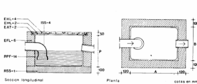
ISS-52 Arqueta sifónica -A-B-P
